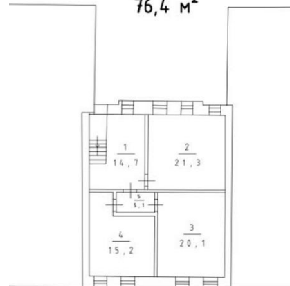
МЕЗОНИН 76,4 м 2
