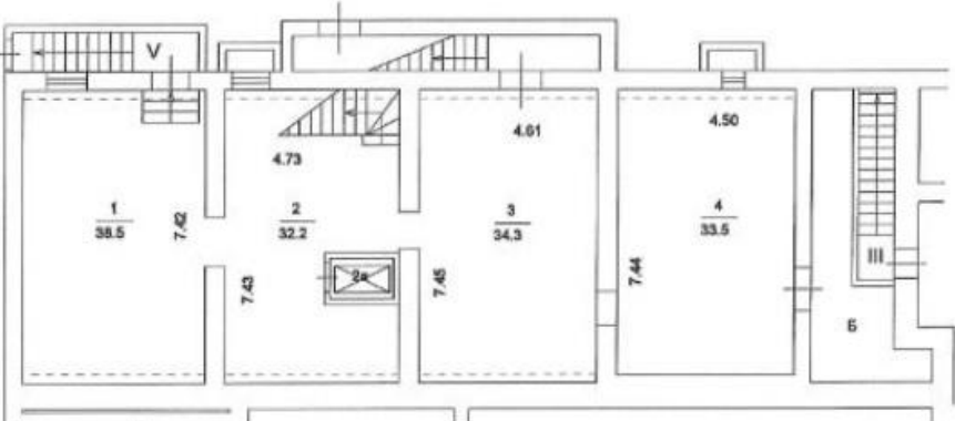
2 ЭТАЖ
