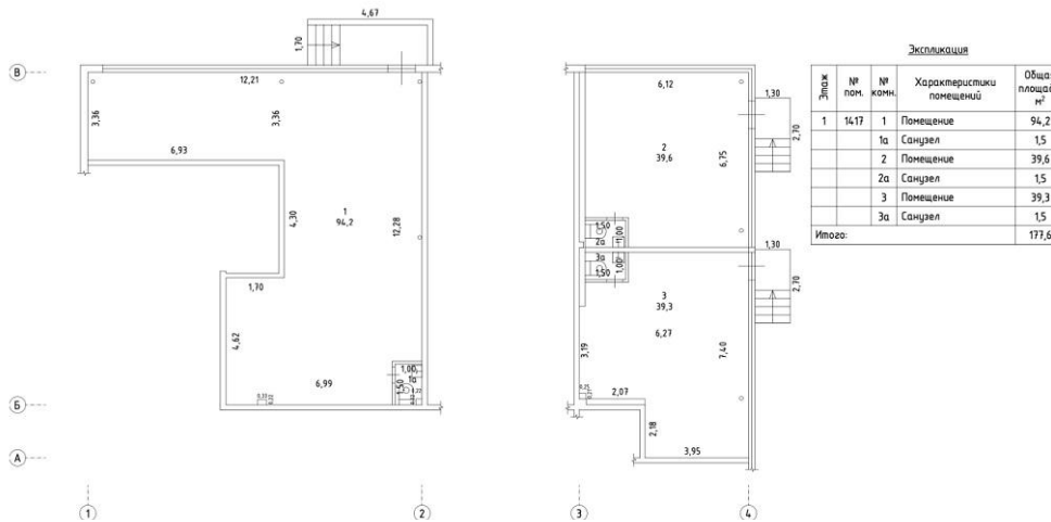
План нежилого помещения после перепланировки М 1:100 1 этаж
