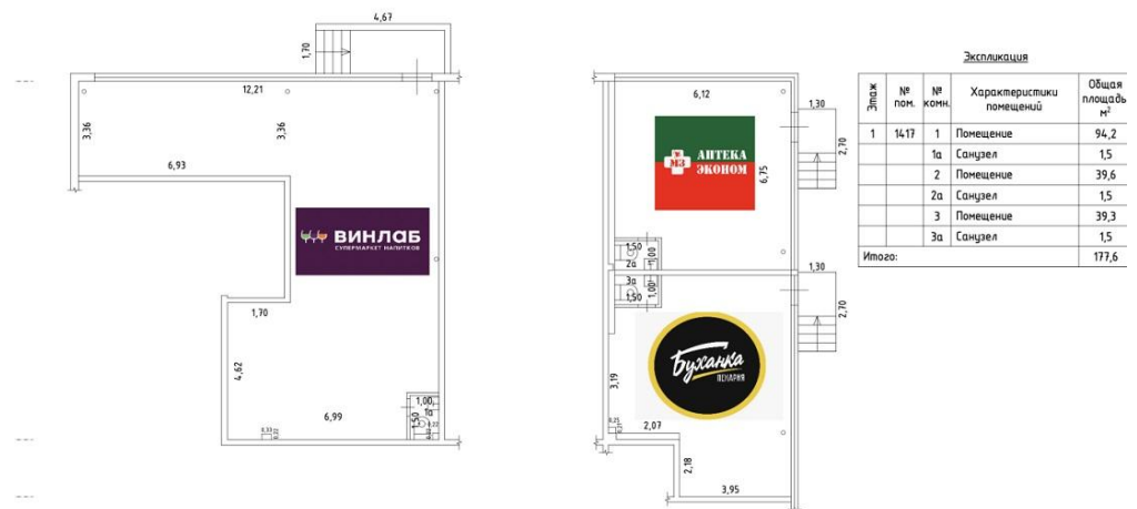
План нежилого помещения после перепланировки М 1:100 1 этаж
