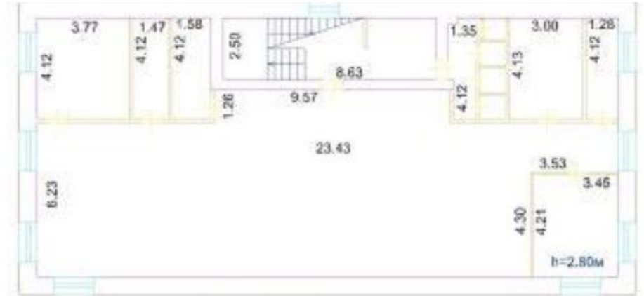
Цокольный этаж
