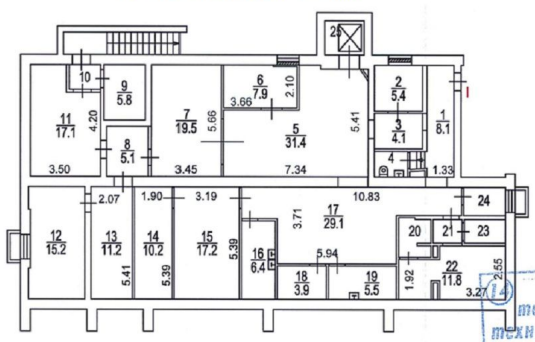
Поэтажный план -1 этаж
