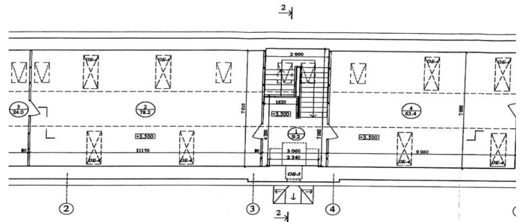
План подкровельного пространства
