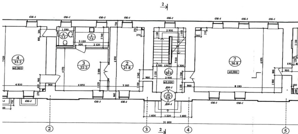
План 1-го этажа
