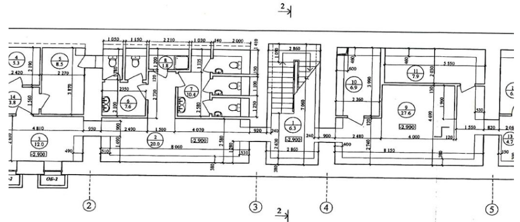
План подвала
